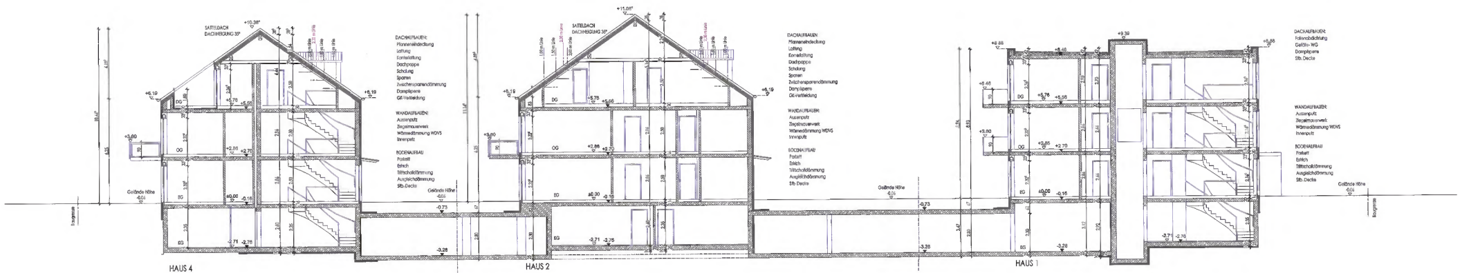
SCHNITT AA
