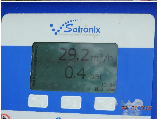
Pumpversuch am 09.07.2020
