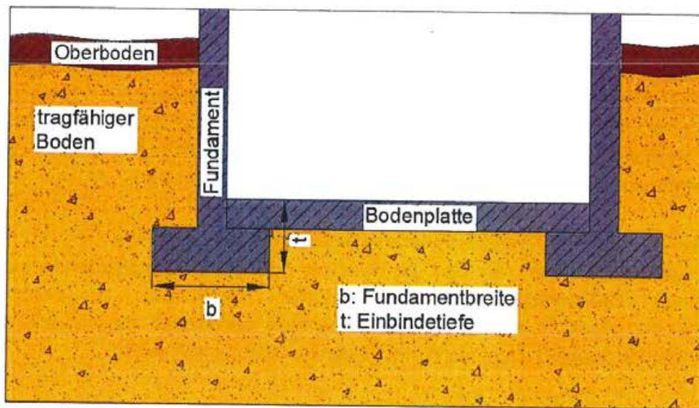
Abbildung 2: Maßgebende Einbindetiefe
