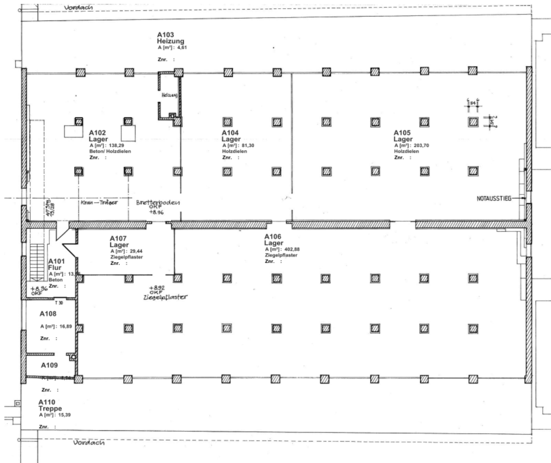
Abb. 3 Grundriss OG
