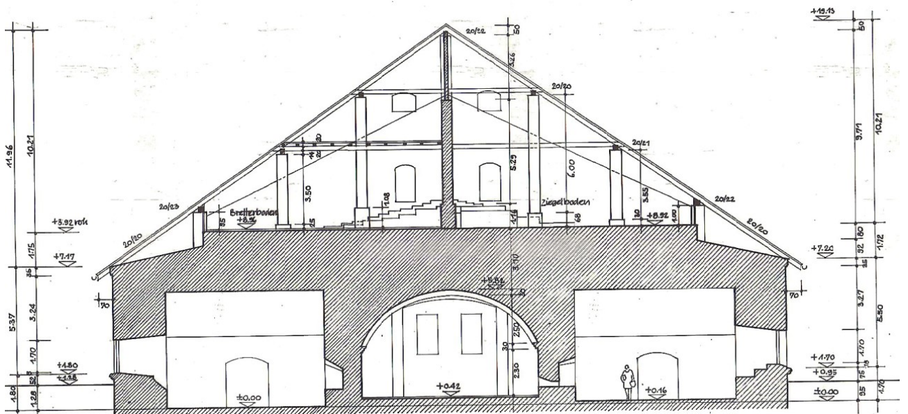
Abb. 2 Querschnitt
