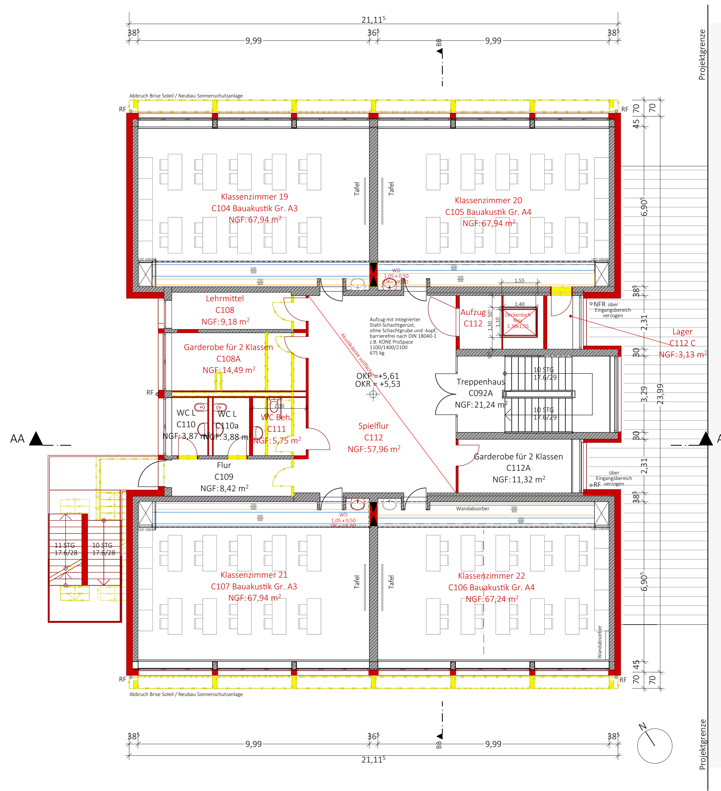
Grundriss 1.Obergeschoss
