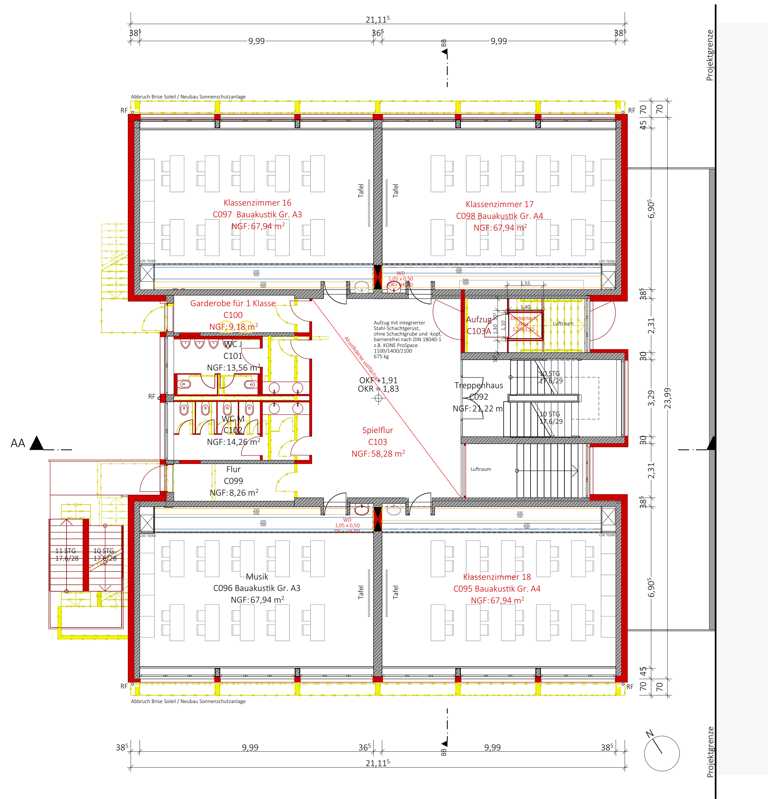
Grundriss Erdgeschoss (Hochpaterre)
