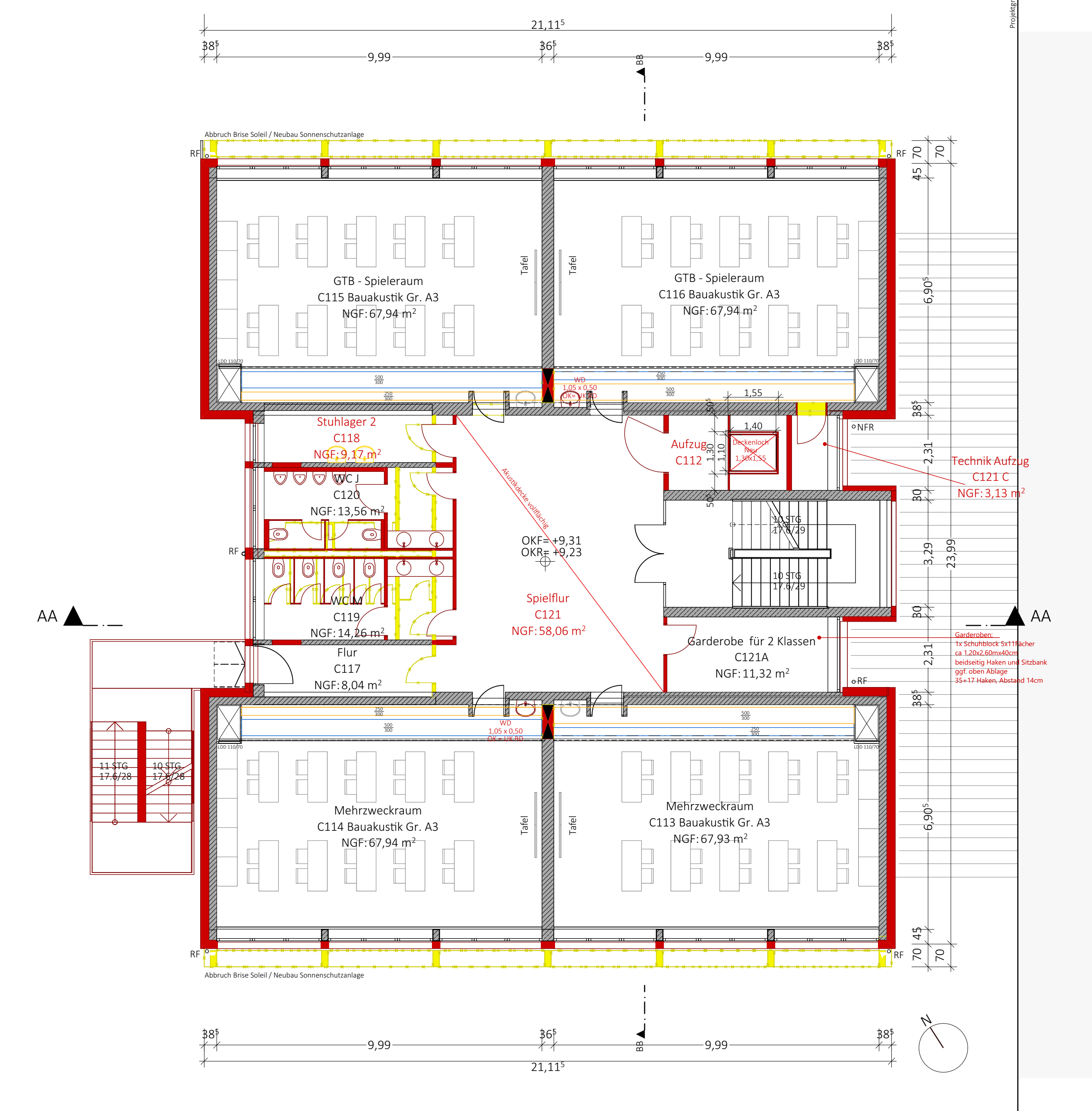
Grundriss 2. Obergeschoss
