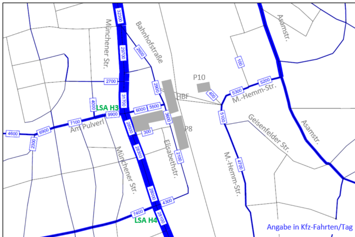
Abbildung 4 Verkehrsmengen Prognose-Nullfall 2035
