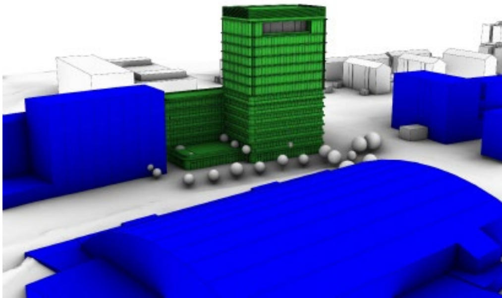
Abbildung 4. Modell des Bauvorhabens (grün) mit Bestandsgebäuden in der Nachbarschaft (blau) – Ansicht aus Nordwest.
