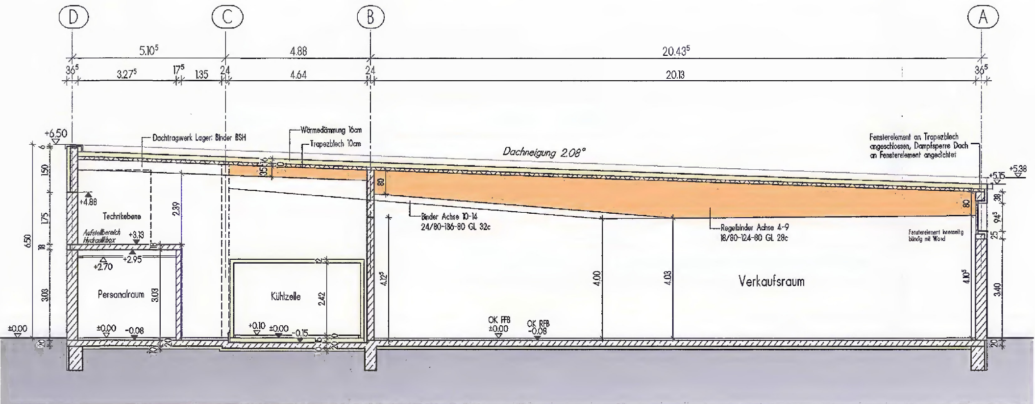
SCHNITT A-A
