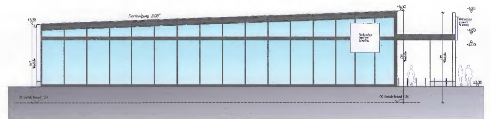
ANSICHT NORD
