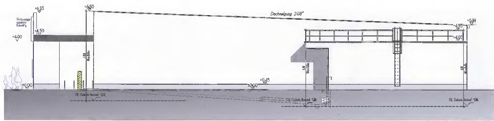
ANSICHT SUD
