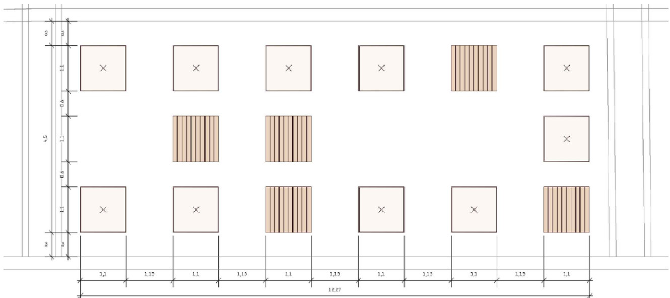
GRUNDRISS
