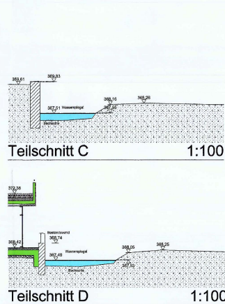
B Schnitt 1:100
