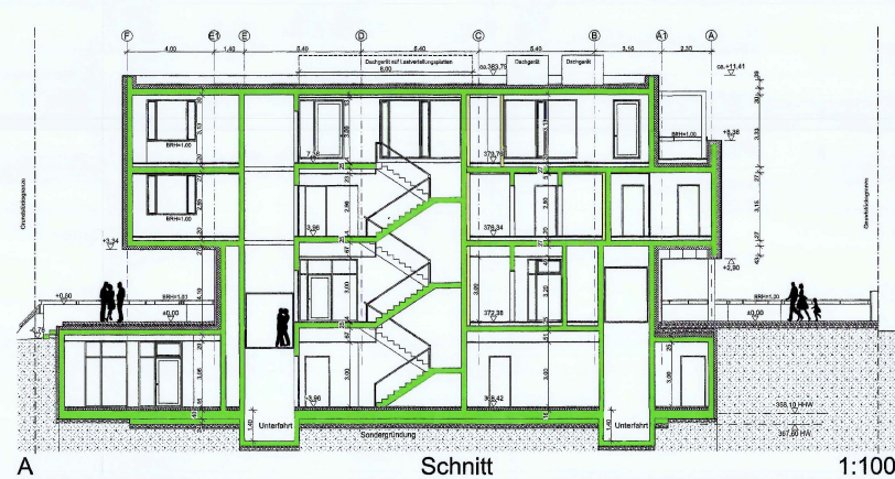
Teilschnitt F 1:100
