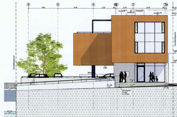
Ost Ansicht 1:100
