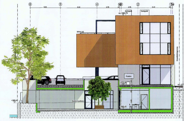
Teilschnitt E 1:100
