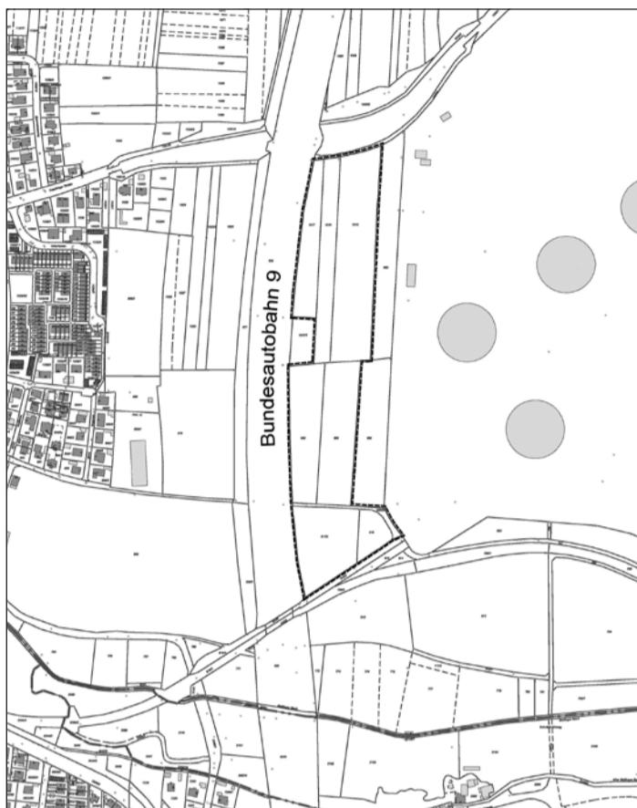
Lageplan zum vorhabenbezogenen Bebauungs- und Grünordnungsplan Nr. 616 „Freiflächenphotovoltaikanlage östlich der BAB 9“ und zur Änderung des Flächennutzungsplanes im Rahmen eines Parallelverfahrens
