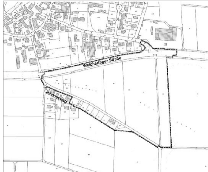
Lageplan zum Bebauungs- und Grünordnungsplan Nr. 904 „Hagau – Am Kirchsteig“
