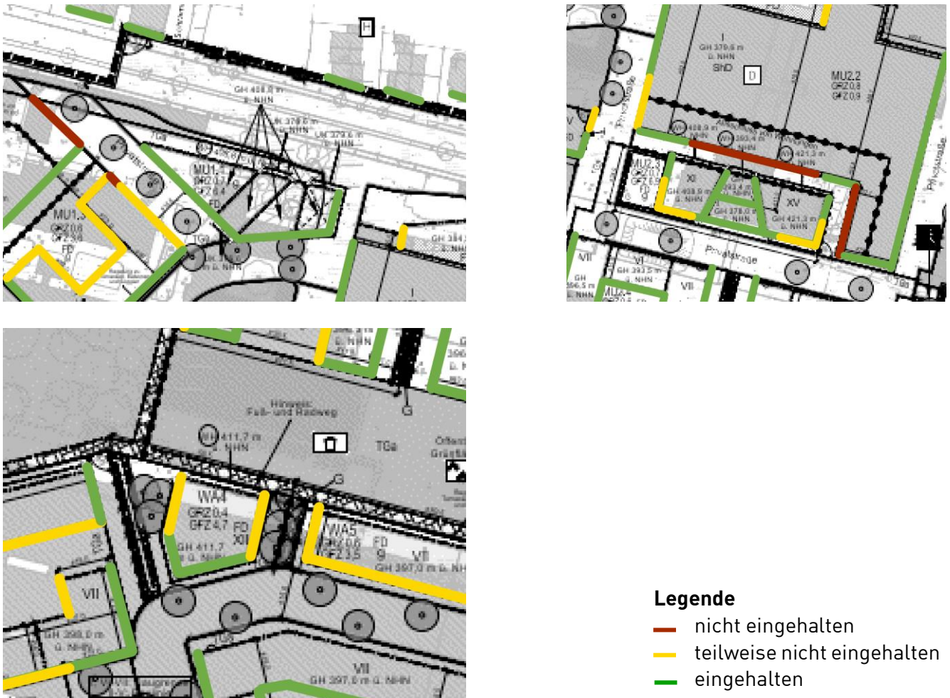
Abbildung 6.15: Übersicht Ergebnisse der Besonnungszeit Baufeld MU 1.1, MU 2.3 und WA 4
