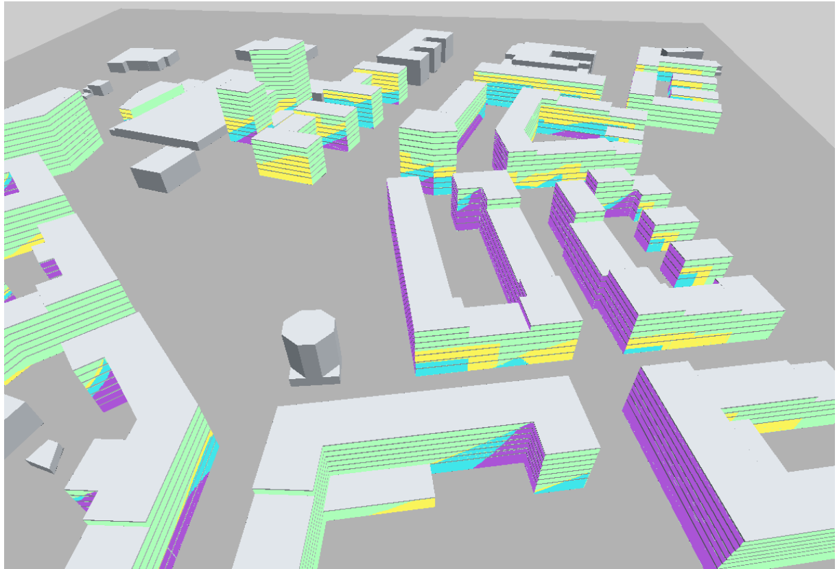
Abbildung 6.8: Verschattung INquartier West – Detailansicht
