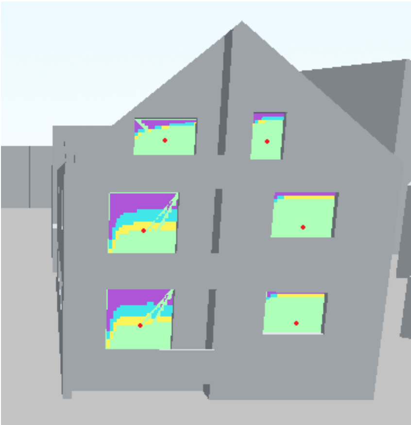
Abbildung 42: Friedrich-Ebert-Straße 74 - 74 1/2, Süd, Nullfall
