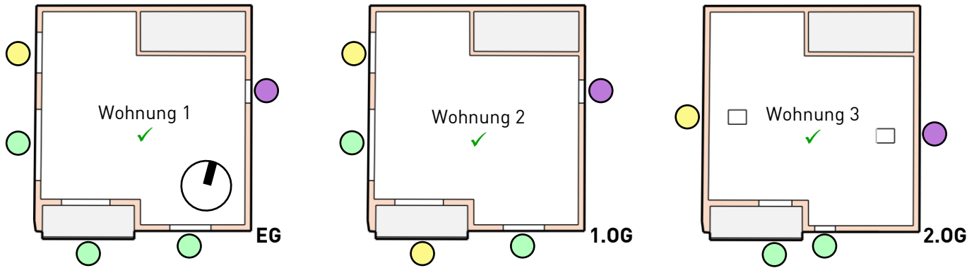
Abbildung 66: Skizze Grundrisse (FES 74 1/3), Nullfall, Grundlage: Bestandspläne
