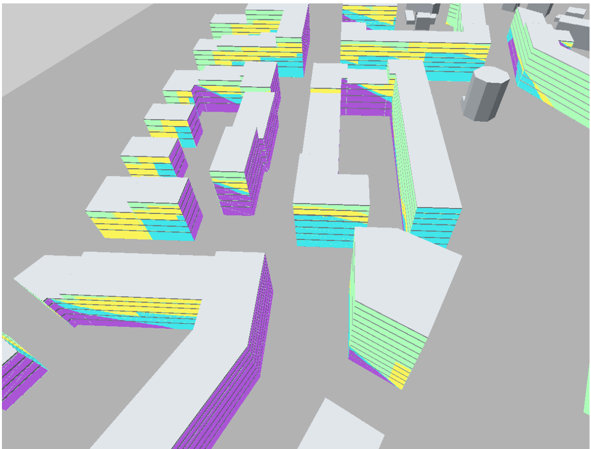
Abbildung 6.3: Verschattung INquartier Ost - Detailansicht
