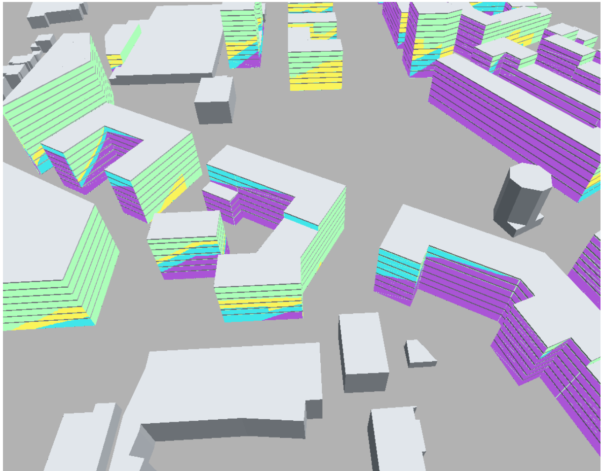
Abbildung 6.11: Verschattung INquartier Nord-West – Detailansicht
