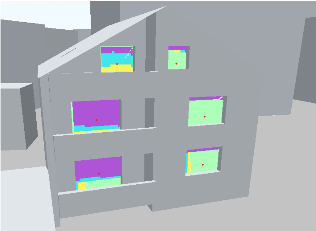
Abbildung 50: Friedrich-Ebert-Straße 74 1/3, Süd, Nullfall
