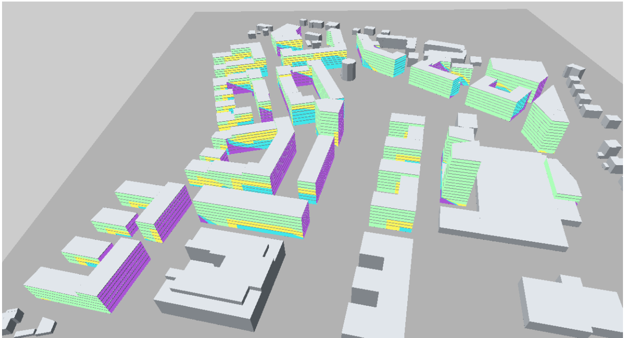
Abbildung 6.2: Verschattung INquartier Ost
