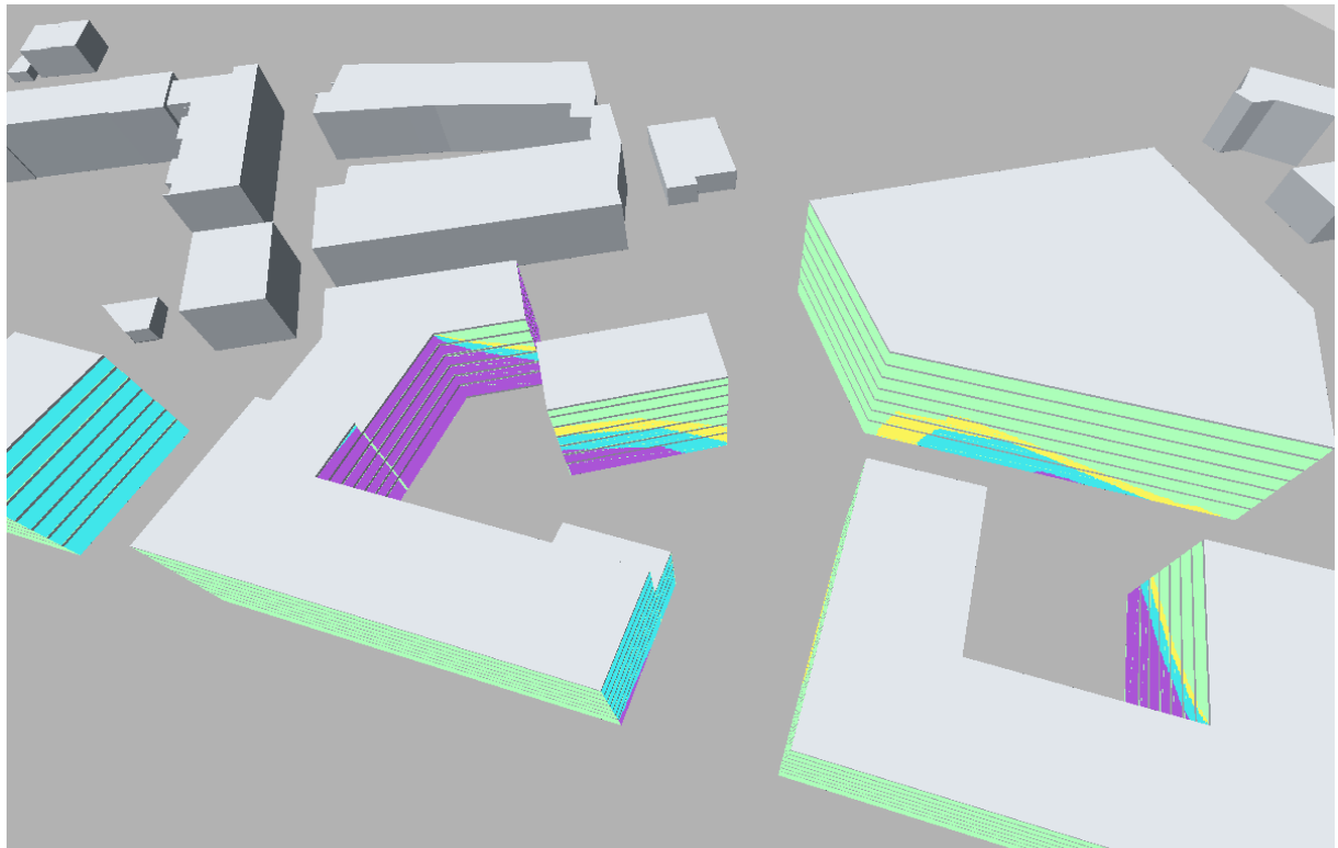
Abbildung 6.4: Verschattung INquartier Nord-Ost – Detailansicht
