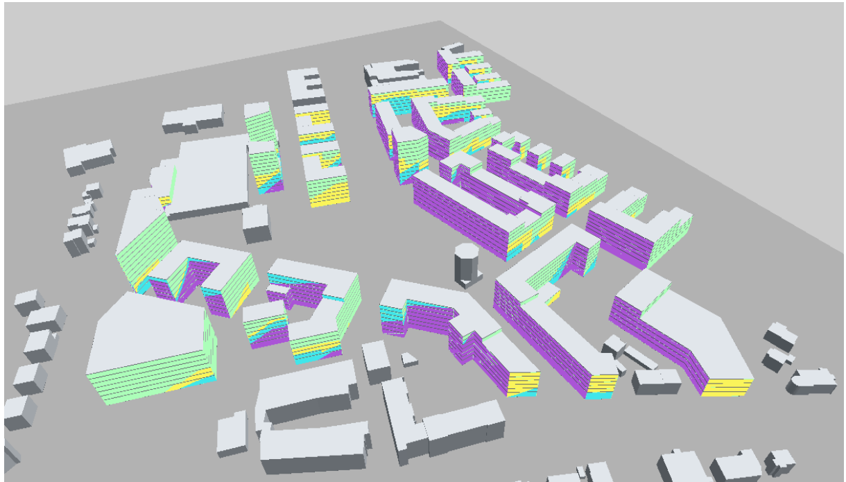
Abbildung 6.10: Verschattung INquartier Nord-West
