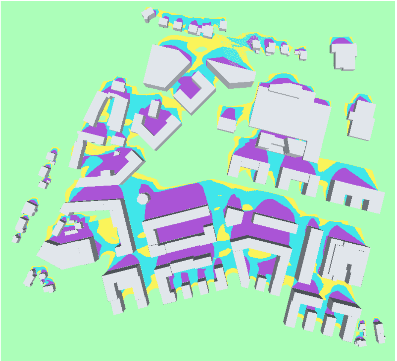
Abbildung 6.14: Verschattung INquartier Aufsicht
