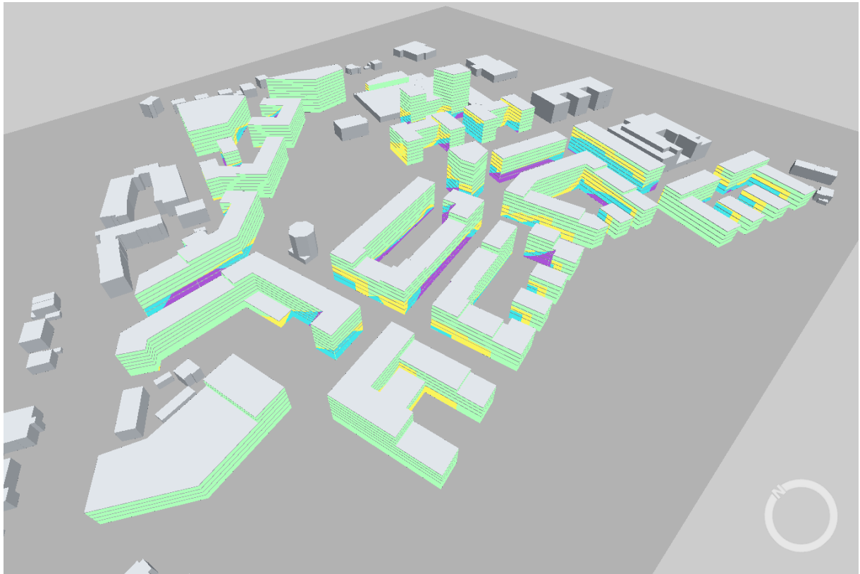
Abbildung 6.6: Verschattung INquartier Süd-West
