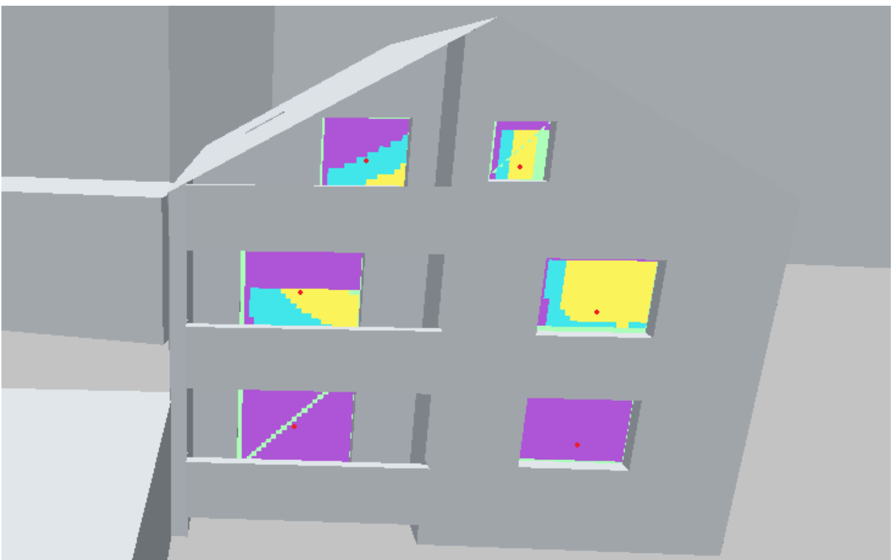
Abbildung 53: Friedrich-Ebert-Straße 74 1/3, Süd, Planstand
