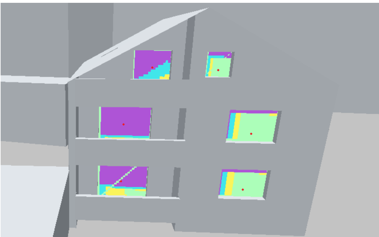
Abbildung 51: Friedrich-Ebert-Straße 74 1/3, Süd, Planstand
