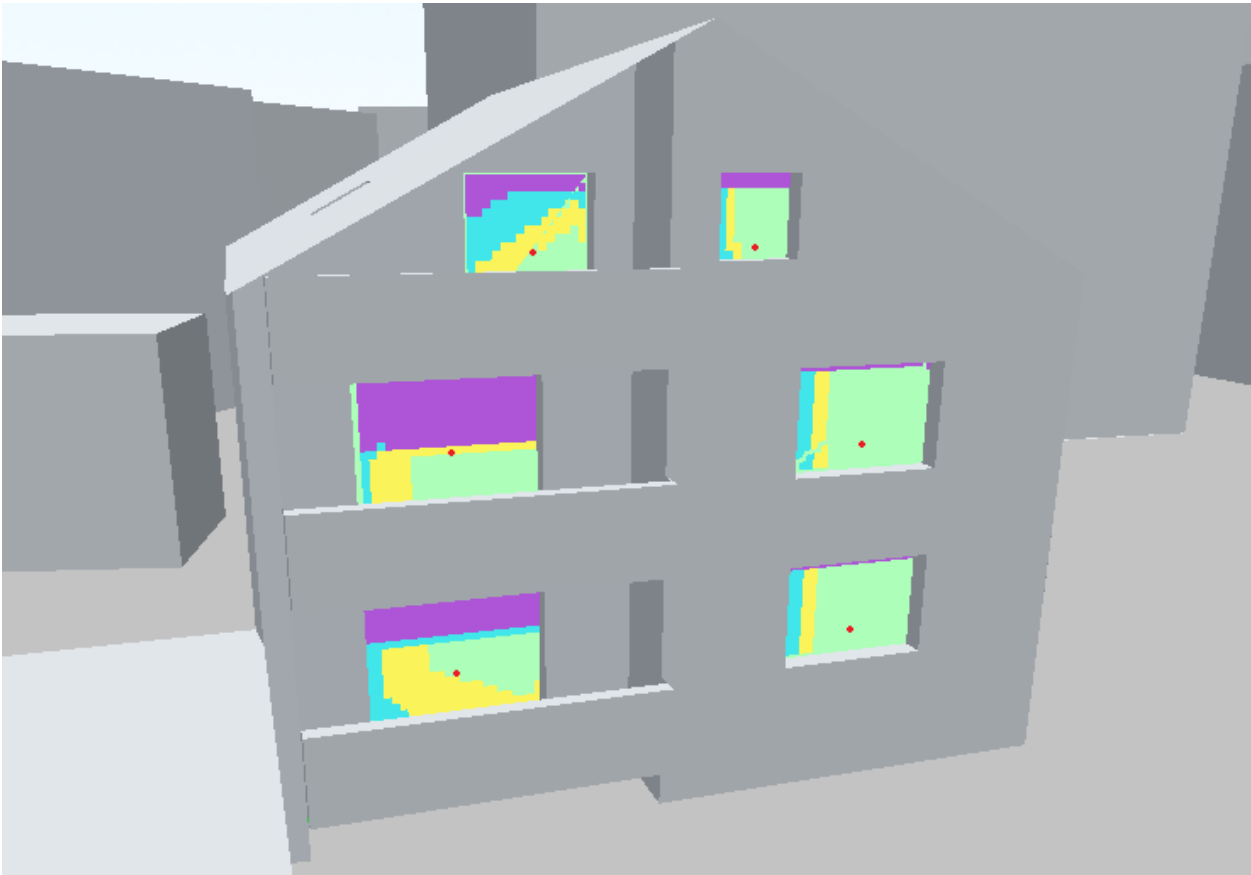
Abbildung 52: Friedrich-Ebert-Straße 74 1/3, Süd, Nullfall
