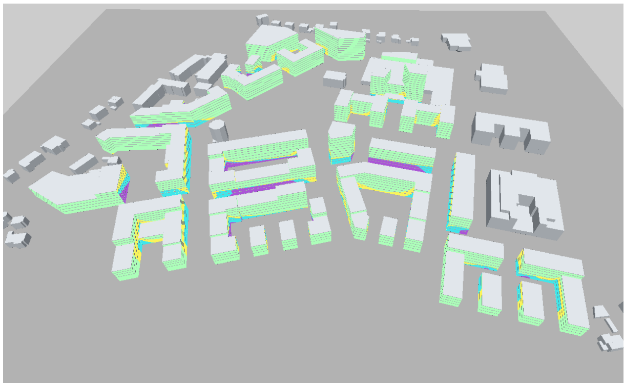
Abbildung 6.1: Verschattung INquartier Süd
