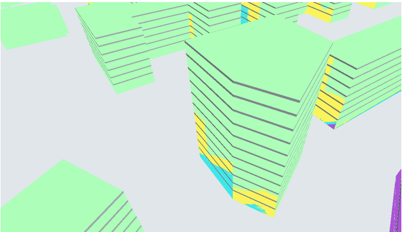
Abbildung 7.17: Verschattung INquartier Detailansicht WA 4 – West
