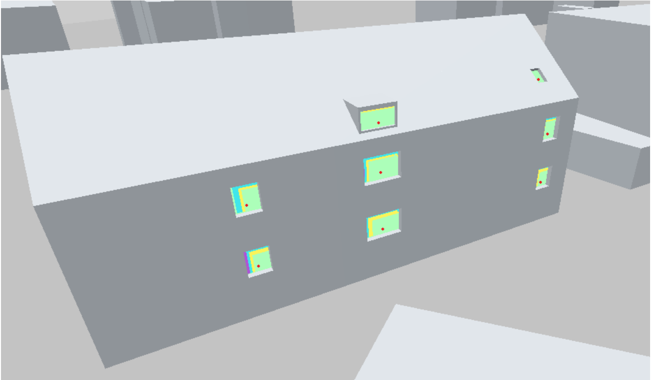
Abbildung 40: Friedrich-Ebert-Straße 74 - 74 1/2, Ost, Nullfall
