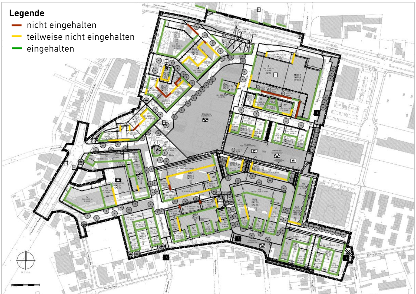
Abbildung 6.21.: Übersicht der Baufelder nach Empfehlungsstufe gering, gem. DIN EN 17037:2022-05
