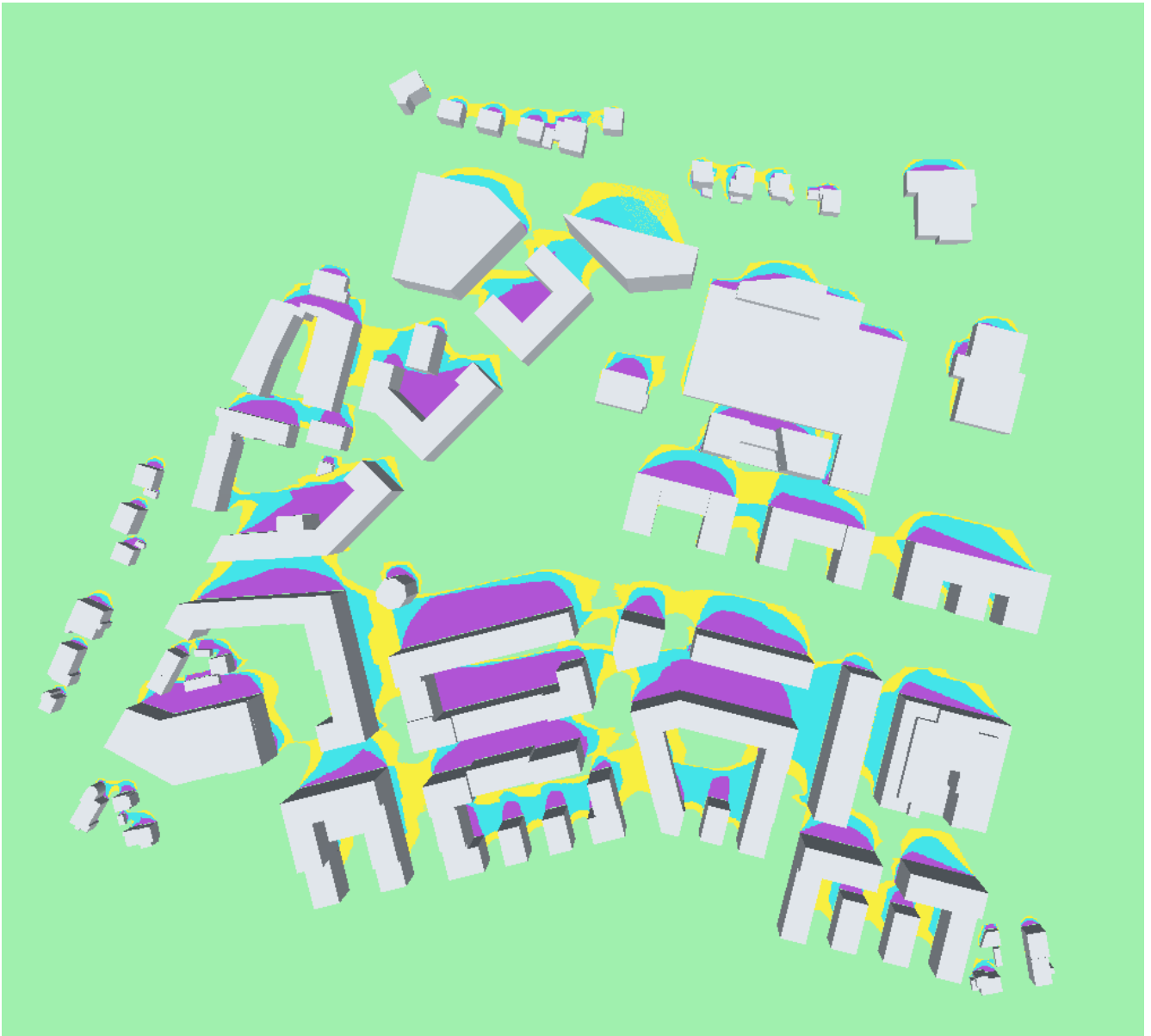
Abbildung 7.12: Verschattung INquartier Aufsicht
