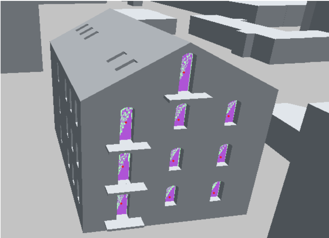
Abbildung 62: Friedrich-Ebert-Straße 80 1/3, West, Nullfall
