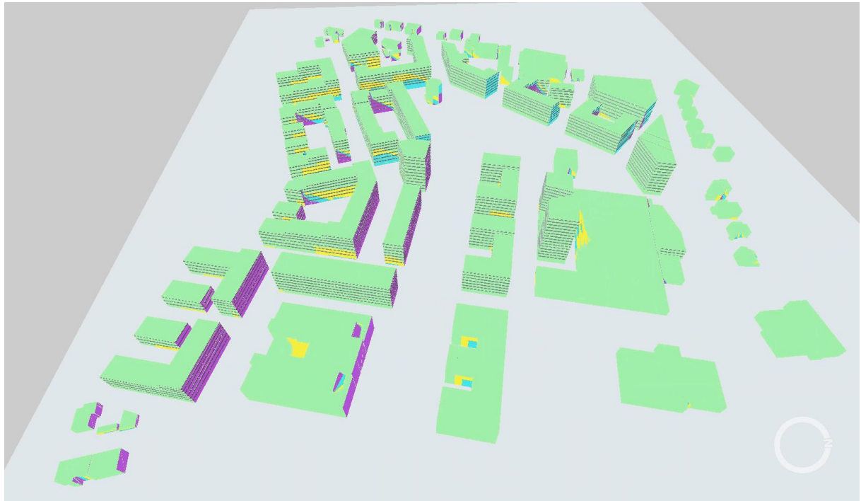
Abbildung 7.2: Verschattung INquartier Ost
