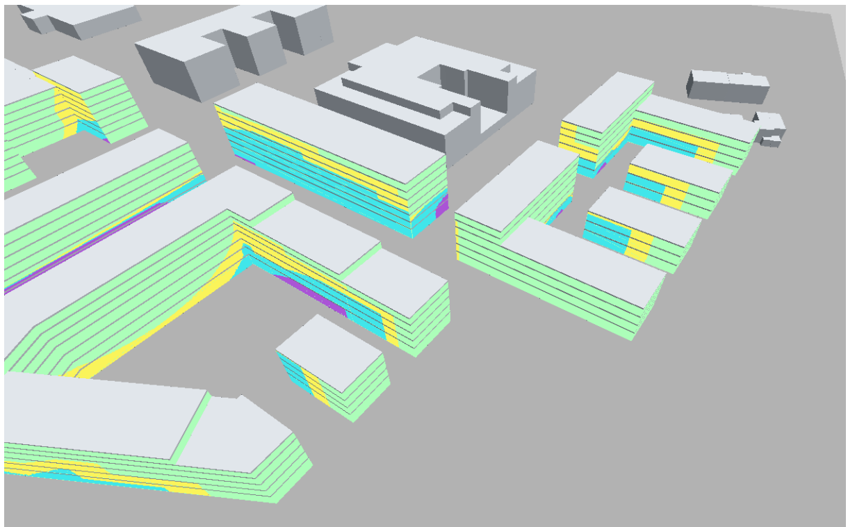
Abbildung 6.7: Verschattung INquartier Süd-West – Detailansicht
