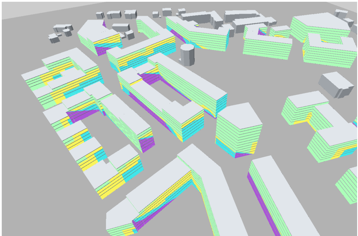
Abbildung 6.5: Verschattung INquartier Süd-Ost
