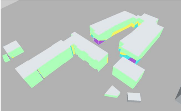
Abbildung 6.29: Friedrich-Ebert-Straße 80-90, Süd, Nullfall
