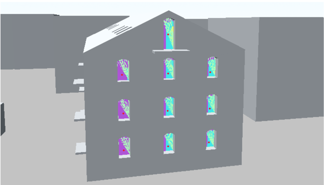
Abbildung 57: Friedrich-Ebert-Straße 80 1/3, Ost, Planstand
