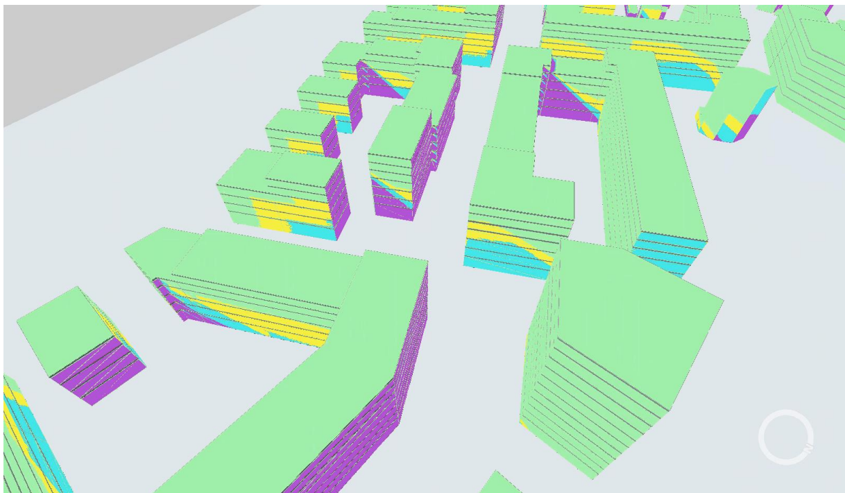
Abbildung 7.3: Verschattung INquartier Ost - Detailansicht
