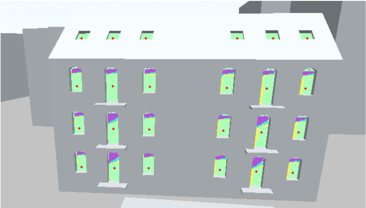
Abbildung 61: Friedrich-Ebert-Straße 80 1/3, Süd, Planstand
