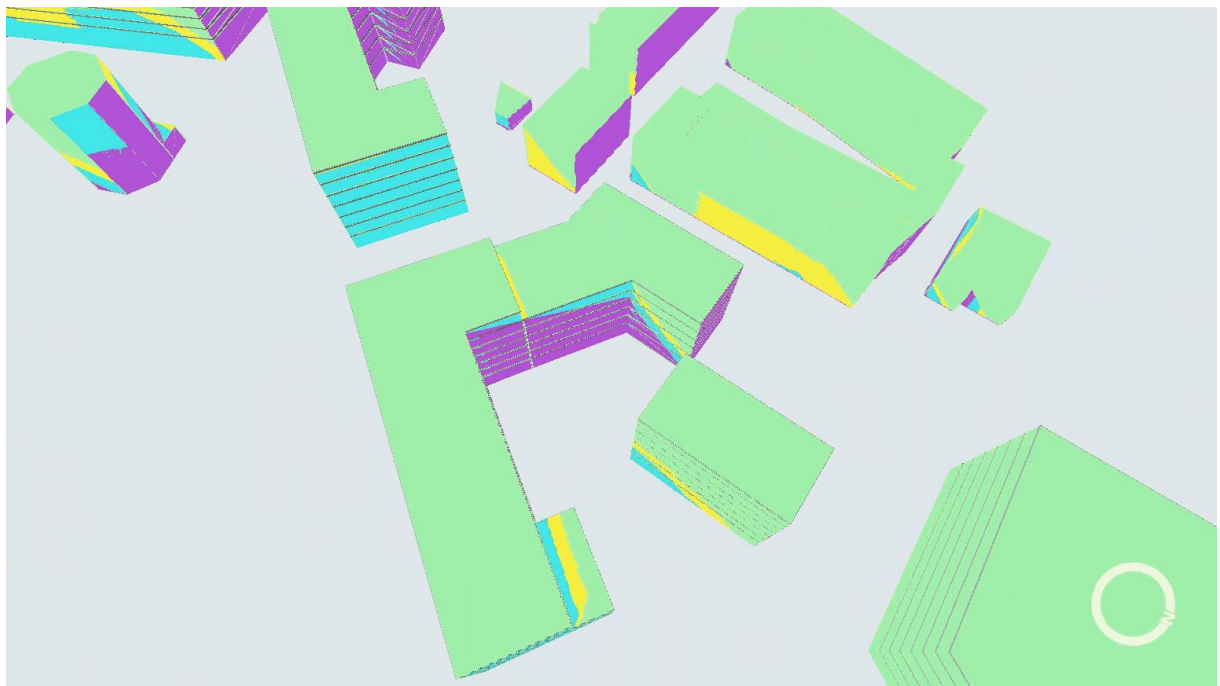
Abbildung 7.11: Verschattung INquartier Nord-Ost – Detailansicht
