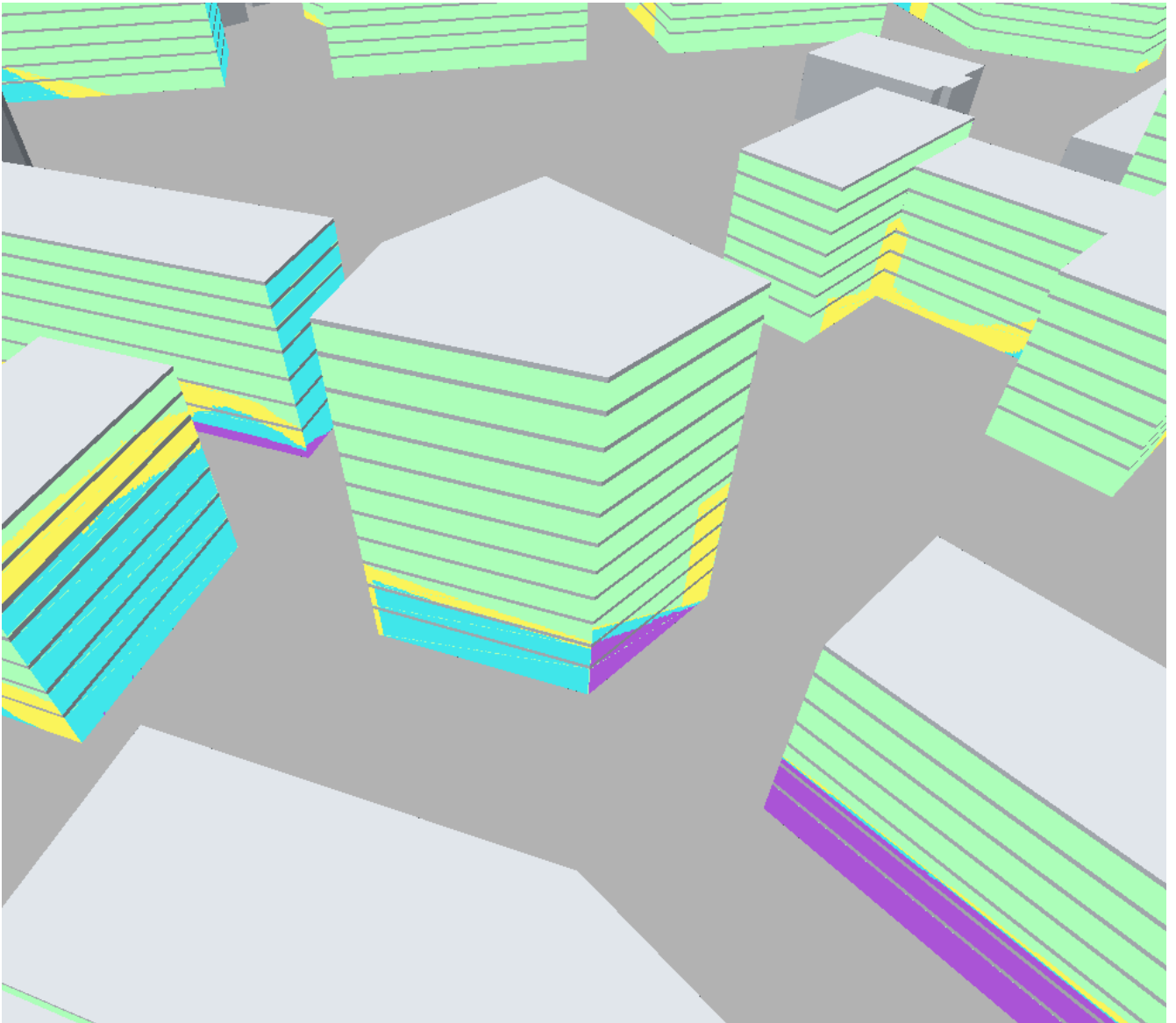
Abbildung 6.20: Verschattung INquartier Detailansicht WA 4 – Südost
