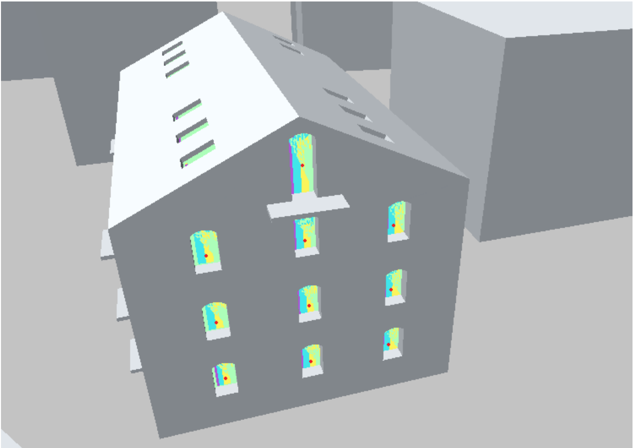
Abbildung 56: Friedrich-Ebert-Straße 80 1/3, Ost, Nullfall
