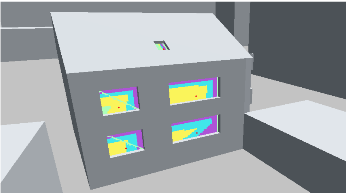
Abbildung 55: Friedrich-Ebert-Straße 74 1/3, West, Planstand
