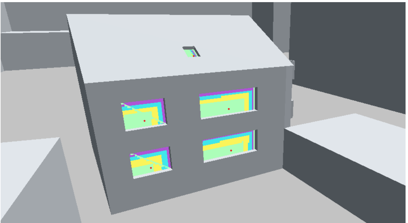
Abbildung 53: Friedrich-Ebert-Straße 74 1/3, West, Planstand
