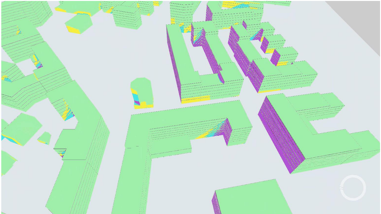
Abbildung 7.8: Verschattung INquartier West – Detailansicht
