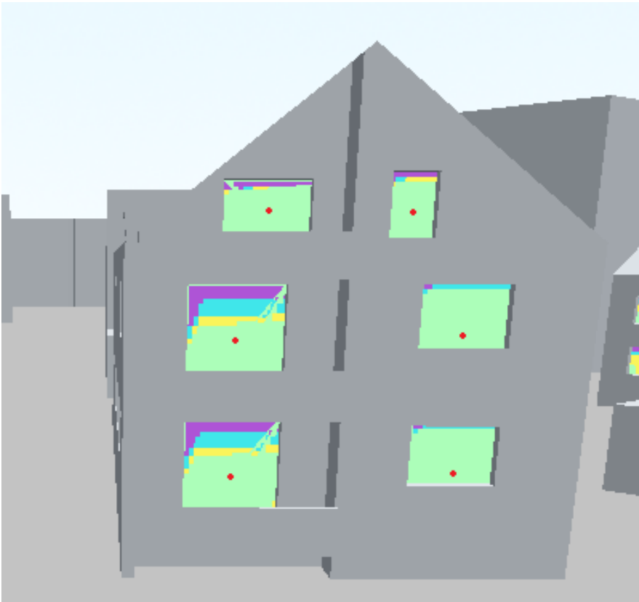
Abbildung 44: Friedrich-Ebert-Straße 74 - 74 1/2, Süd, Nullfall
