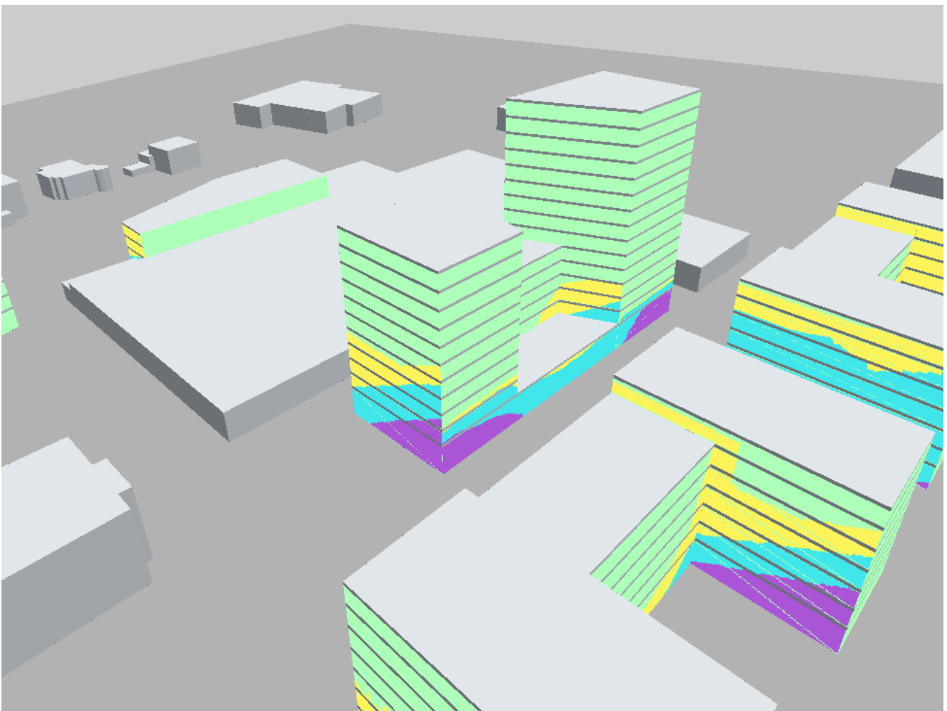
Abbildung 6.17: Verschattung INquartier Detailansicht MU 2.3 – West
