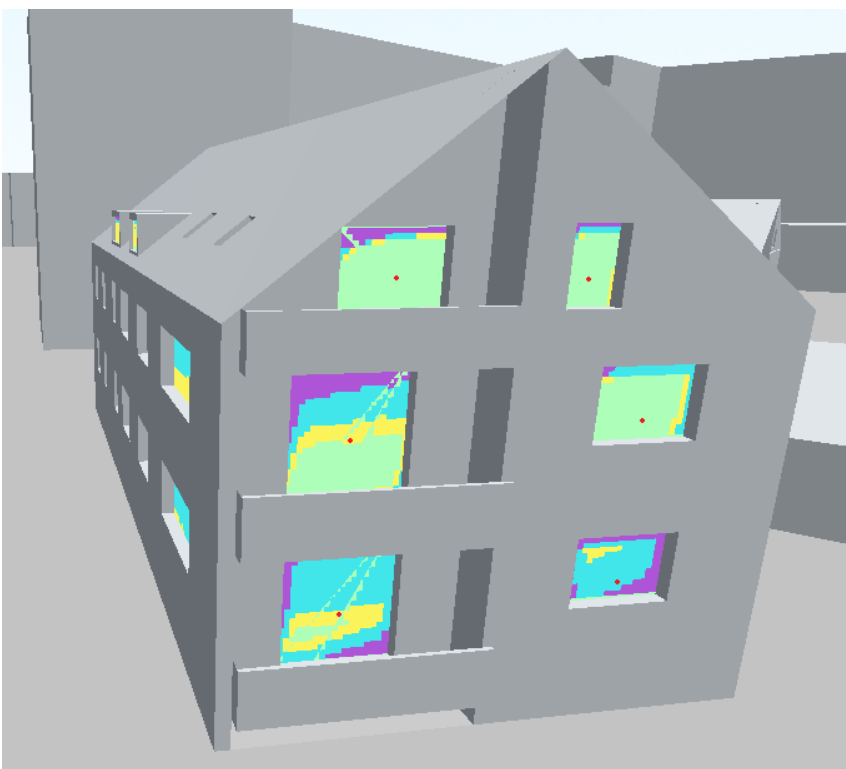
Abbildung 43: Friedrich-Ebert-Straße 74 - 74 1/2, Süd, Planstand
