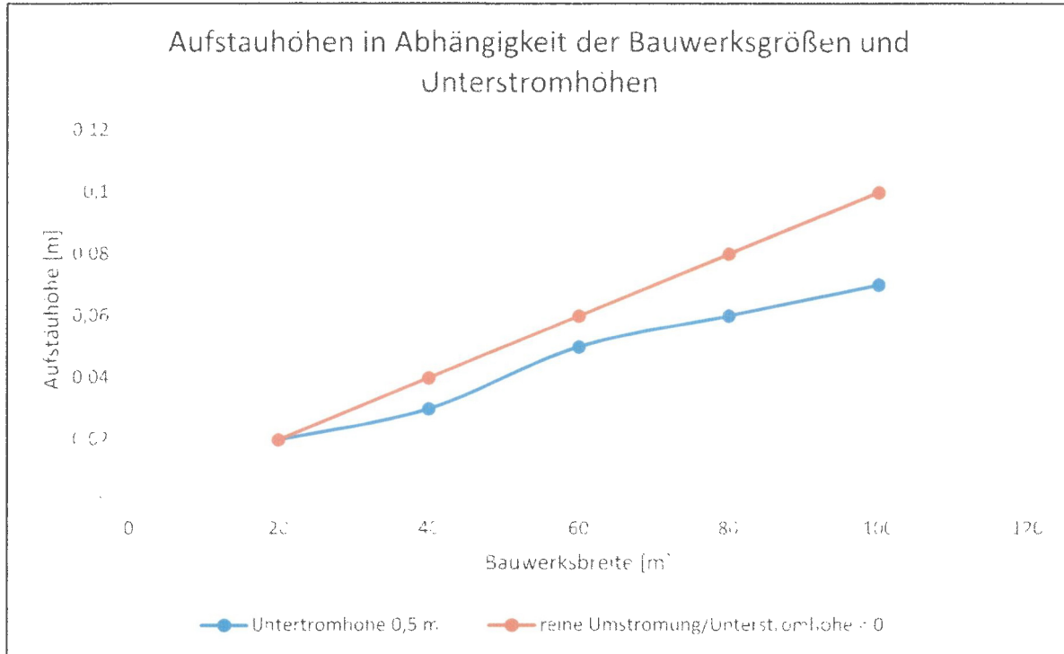
Abb. 1: Nach SCHNEIDER berechnete Aufstauhöhen bei Einbindung der Bauwerkskörper in das Grundwasser. Blaue Linie: Einbindung bis 0,5 m über der Aquifer-sole, orange Linie: komplette Absperrung des Grundwasserstroms ohne Unterströmung (worst case)
