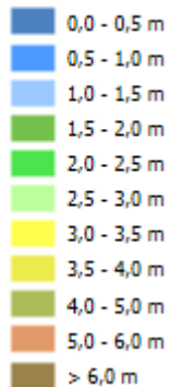
Grundwasserflurabstände für MHGW-Verhältnisse
