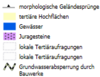
Beeinflussung des Grundwasserkörpers durch geologische Besonderheiten
